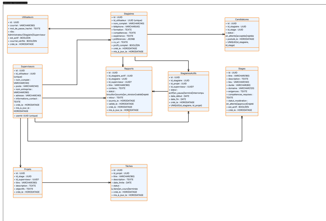
FIGURE V.1 – Figure V.1 : Diagramme de classes UML : entités principales et relations
